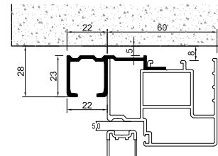
TELAIO CON BINARIO PER GRANDI LUCI
