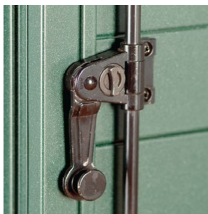
DETTAGLIO GANCIO SPAGNOLETTA DI CHIUSURA.
