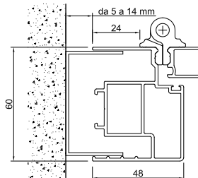
TELAIO TELESCOPICO CON COMPENSATORE A MURO
