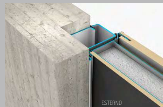
5 Soluzione filomuro esterno senza profili di copertura telaio (Kit posa controtelaio FE)
