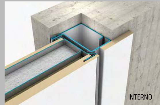
2 Soluzione telaio filomuro con coprifilo piatto per copertura interna (Kit posa controtelaio FI)
